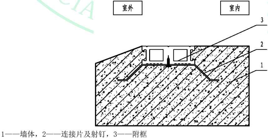
图12 标准化附框前装式构造示意图
