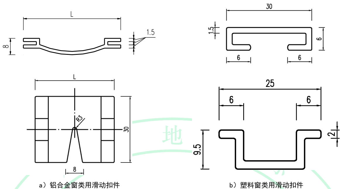
图9 滑动扣件示意图
