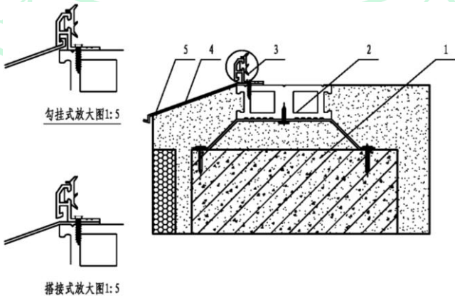
1——墙体，2——附框，3——附框压条，4——披水板，5——密封胶
