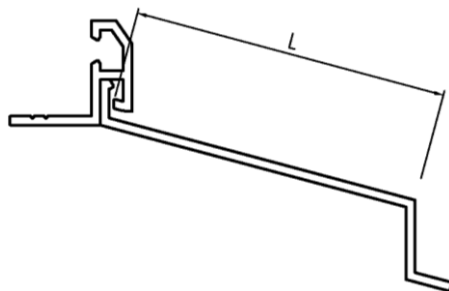
图10 披水板与附框压条连接示意图
