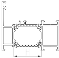
图4 聚酰胺隔热条截面尺寸示意图
