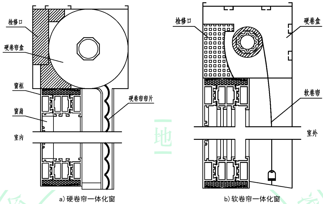
图A.2 外遮阳一体化窗示意图
