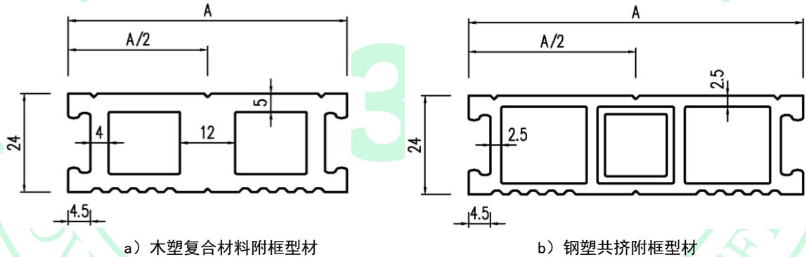
图6 附框型材截面示意图
