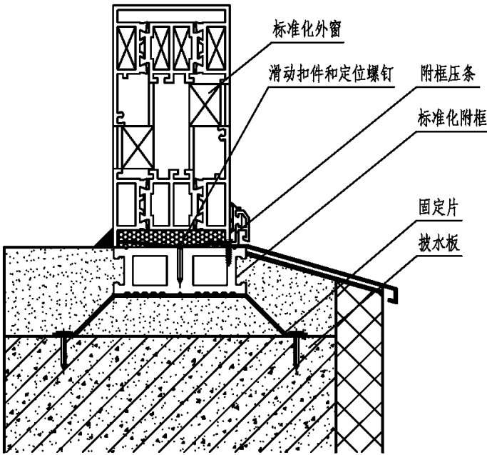
图A.1 标准化外窗系统示意图
