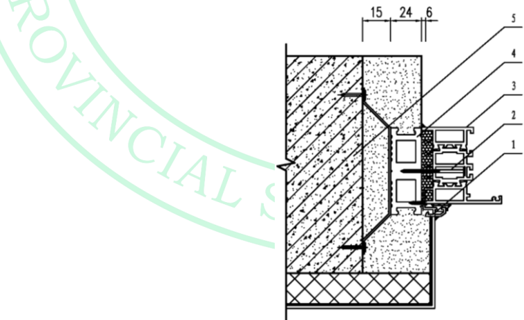
1——附框压条，2——固定螺钉，3——窗框，4——附框，5——墙体
