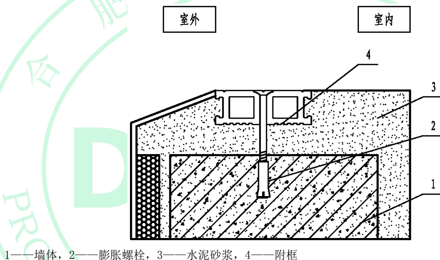
图13 改造居住建筑凹侧面附框安装构造示意图
