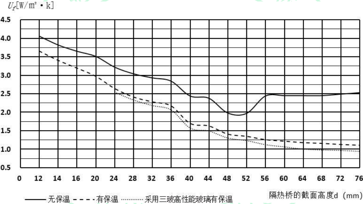
图C. 1 金属窗框采用不同隔热桥截面高度与传热系数关系曲线
