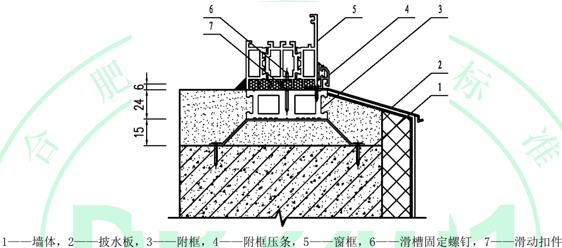
图17 塑料窗下框安装构造示意图
